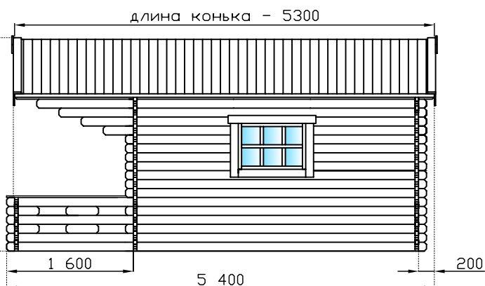
Вид сбоку:
