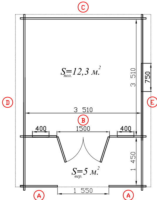
План домика:
